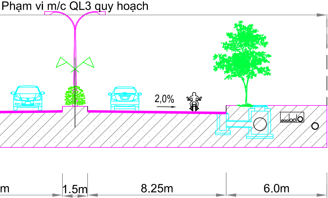
MẶT CẮT QL3
