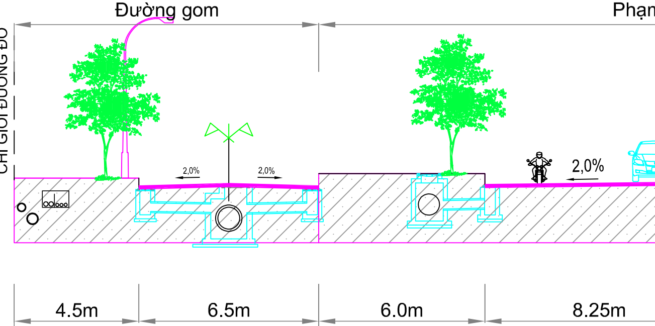
MẶT CẮT 4 - 4
