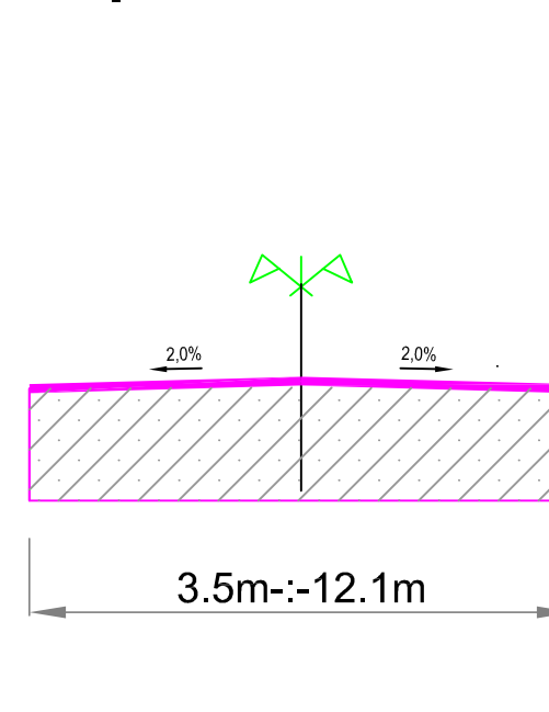
MẶT CẮT 3A - 3A
