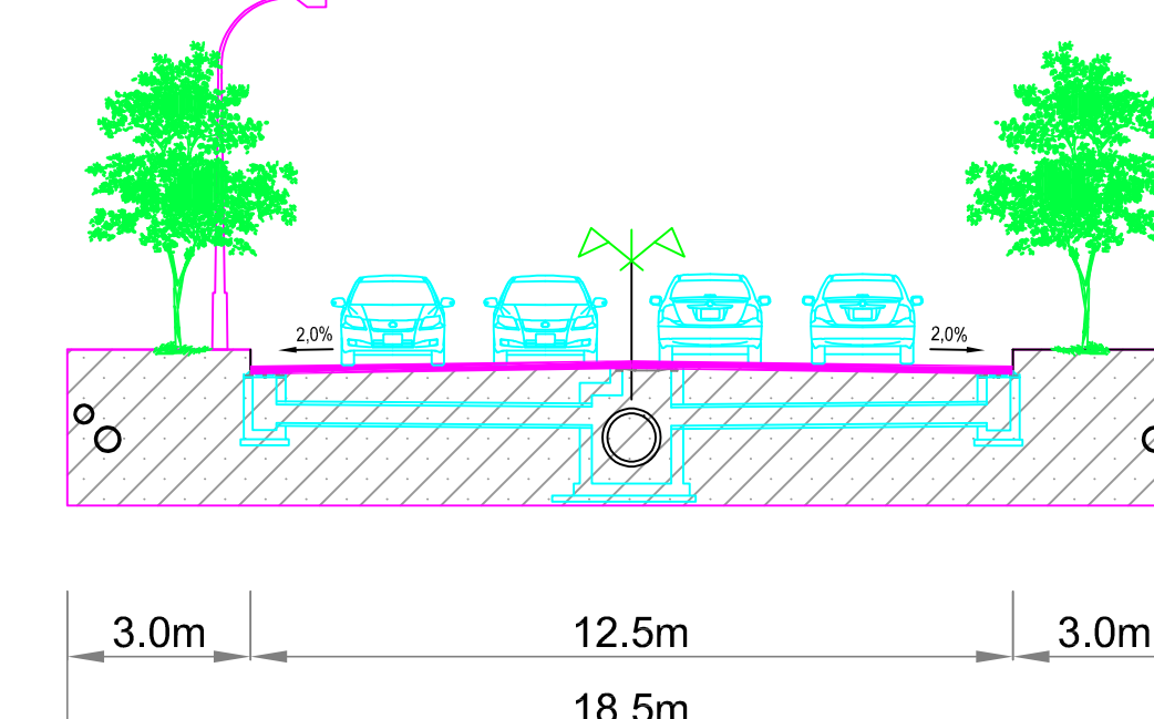
MẶT CẮT 2A - 2A
