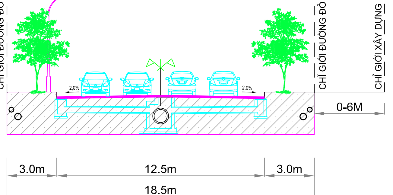
MẶT CẮT 1 - 1
