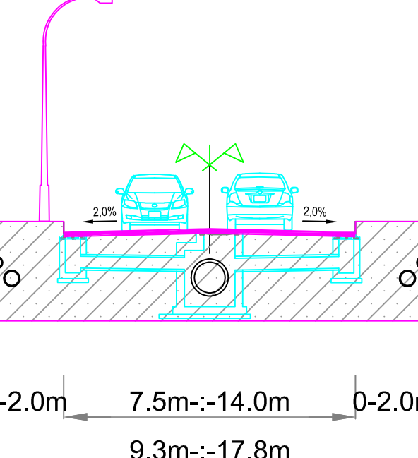
MẶT CẮT 3A - 3A
